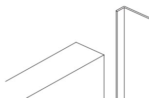
DGPR / S - W - B profilo terminale a L in alluminio L shaped aluminium terminal profile sezione/section 2 x 0,5 cm lunghezza/length: 240-120-60 cm
